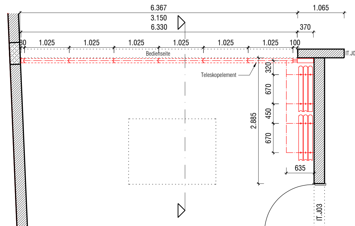
Grundriss 1:50
