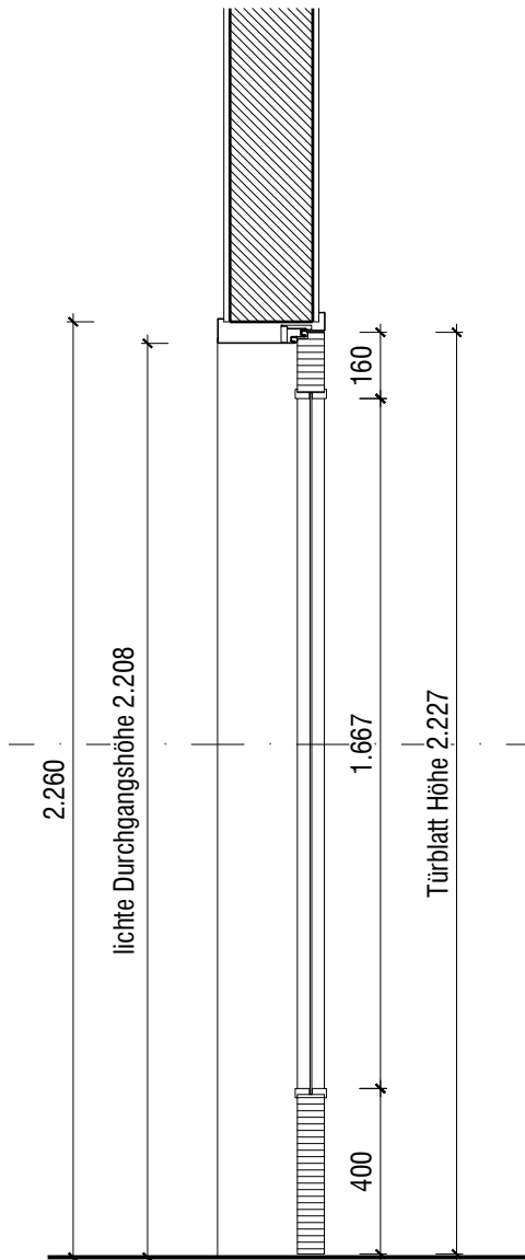
Vertikalschnitt
