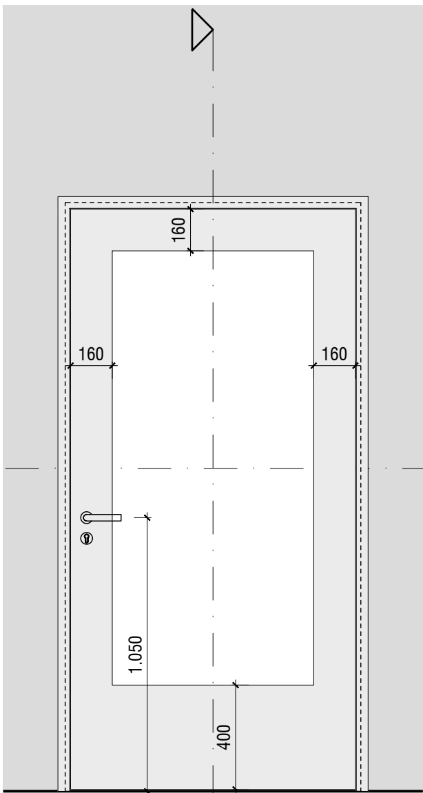
Ansicht Bandseite
