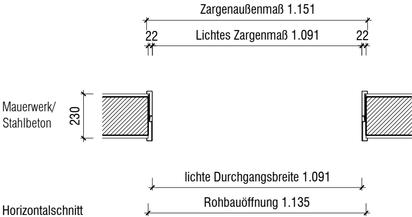
Horizontalschnitt
