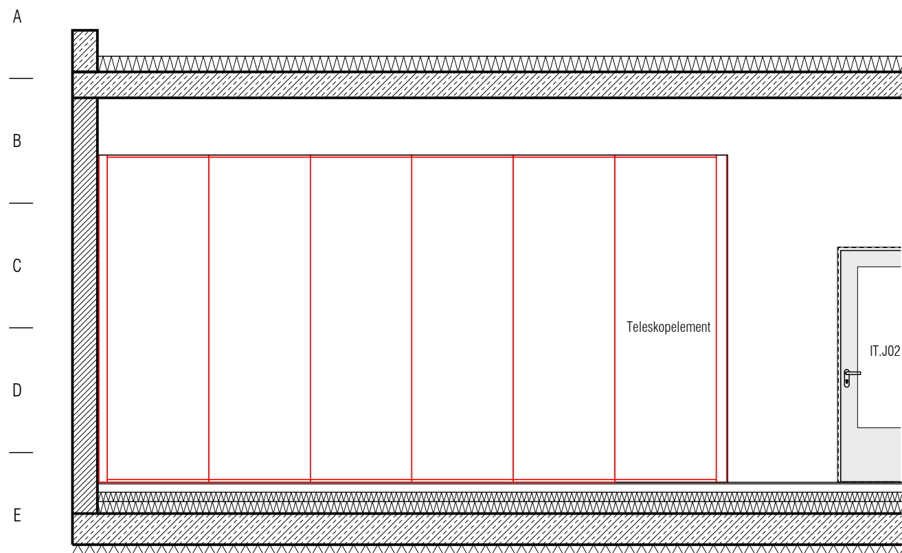
Ansicht Bedienseite 1:50
