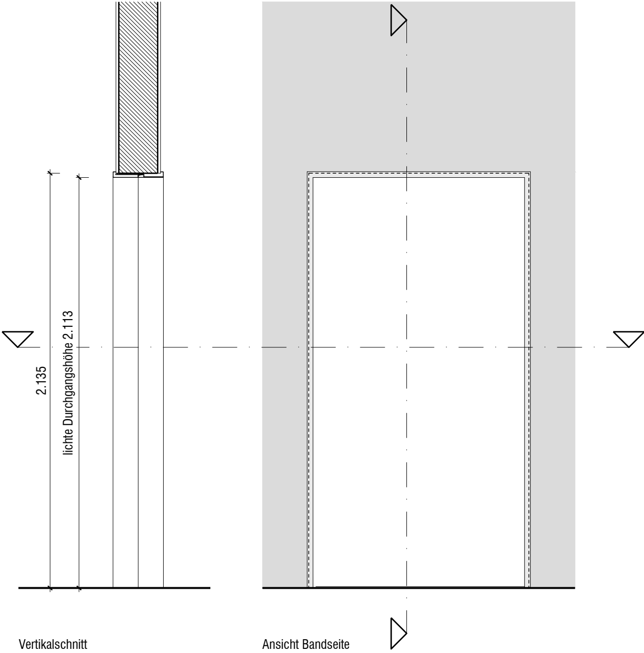
Vertikalschnitt
