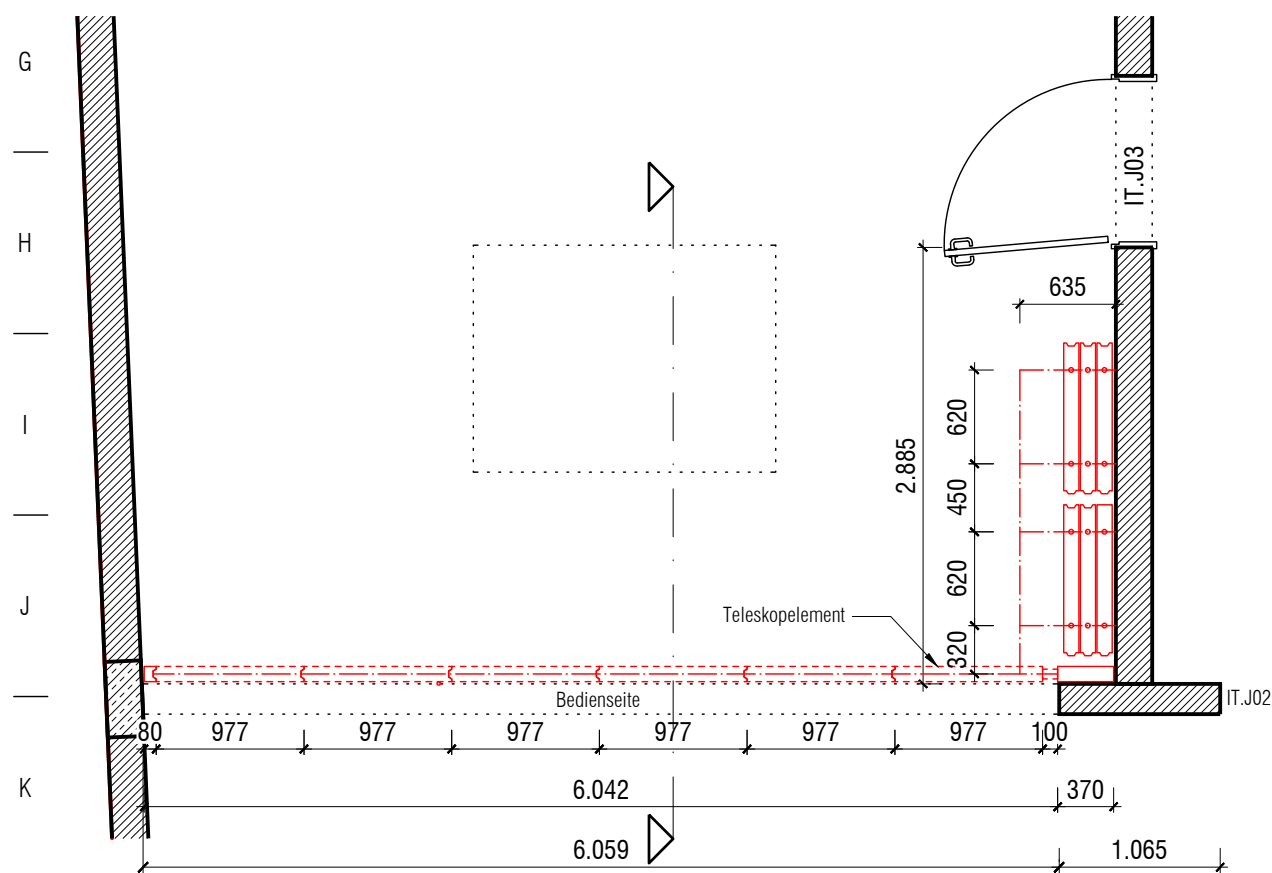
Grundriss 1:50
