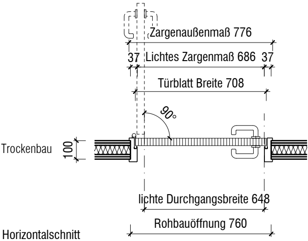
Horizontalschnitt
